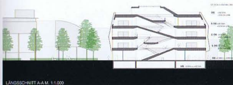
LÄNGSSCHNITT A-A M. 1:1.000
