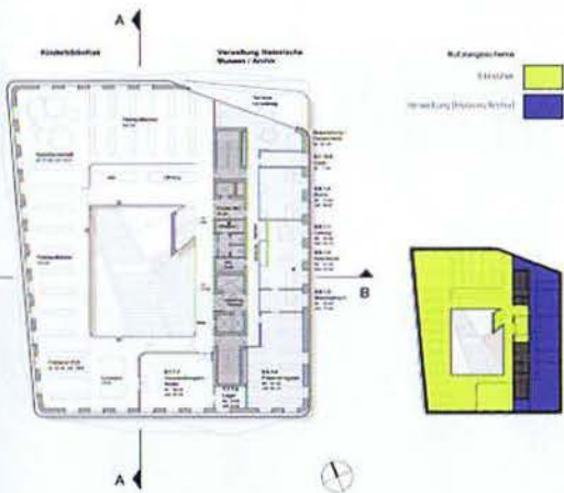
3. OBERGESCHOSS M. 1:1.000
