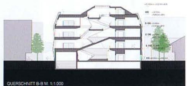
QUERSCHNITT B-B M. 1:1.000
