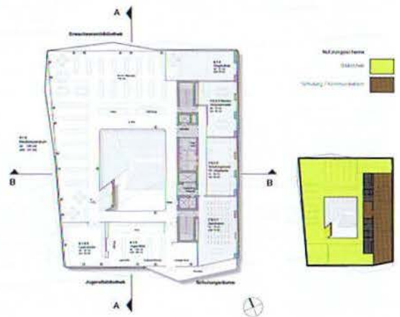
1. OBERGESCHOSS M. 1:1.000
